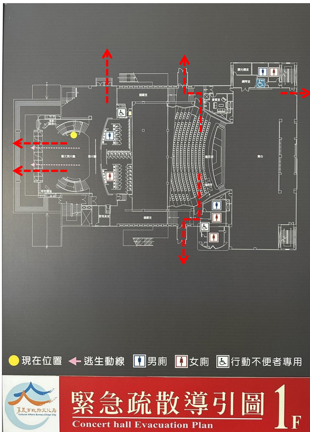
附圖 1-嘉義市政府文化局音樂廳 1F 平面圖暨逃生避難圖
